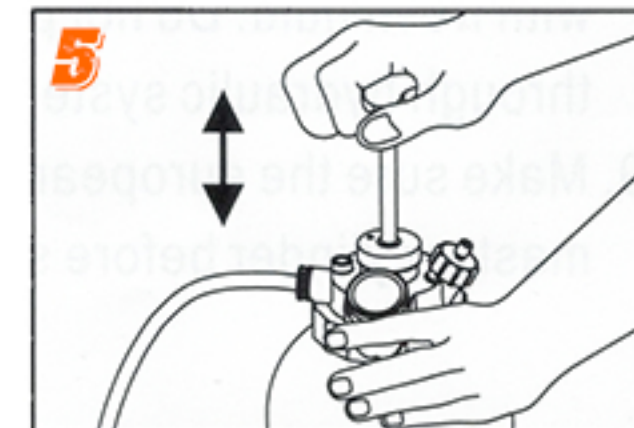
Mise en pression. Dévisser / visser les purgeurs les uns après les autres Pump the handle up and down to discharge the fluid
